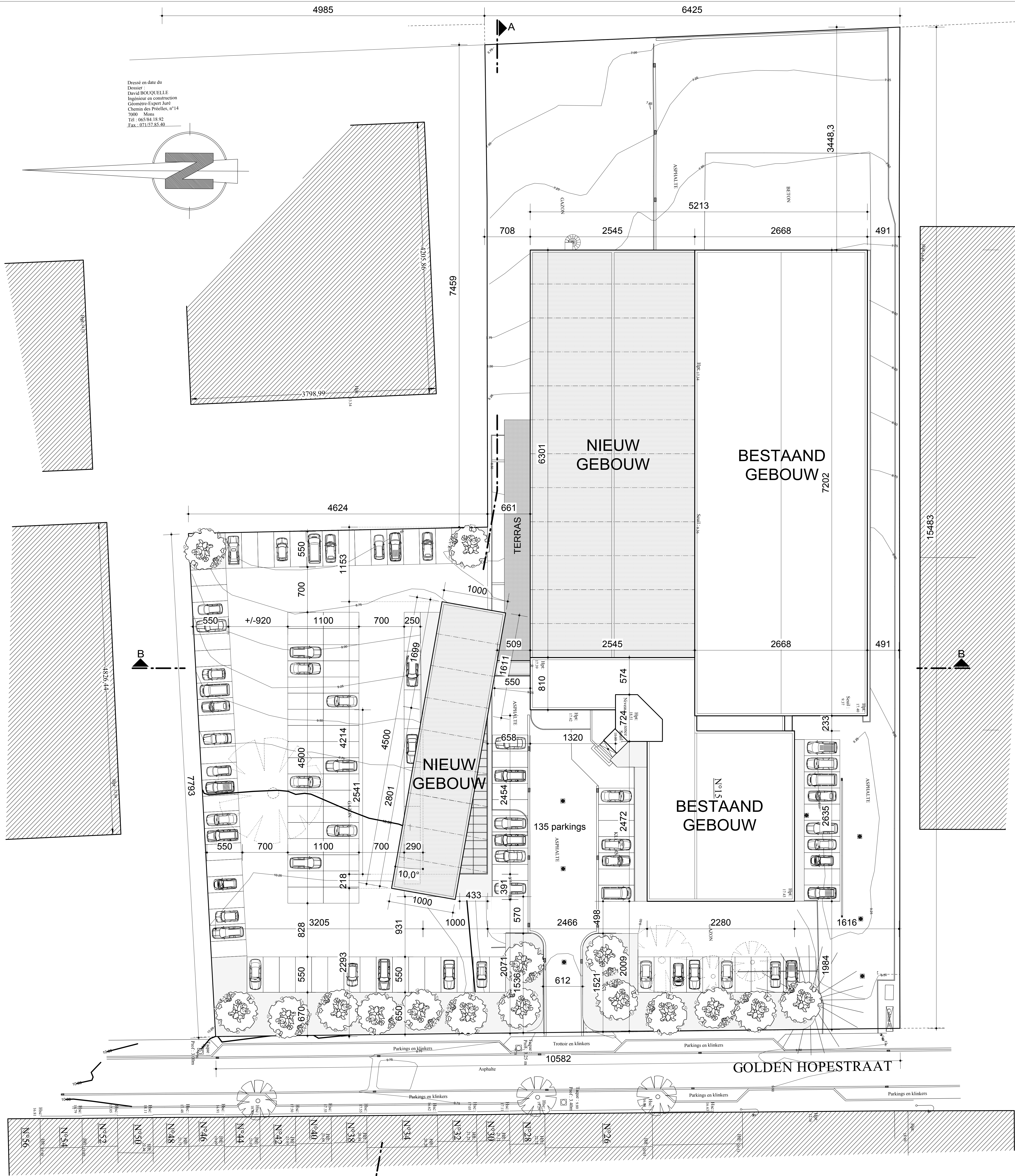
INPLANTINGSPLAN schaal 1/250
