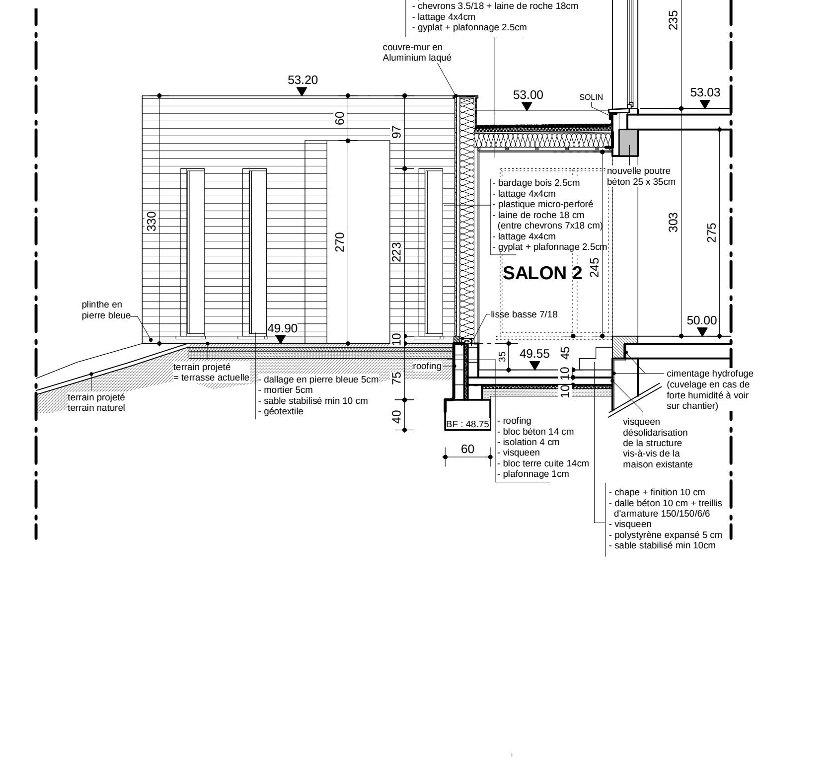
COUPE CC 1/50
