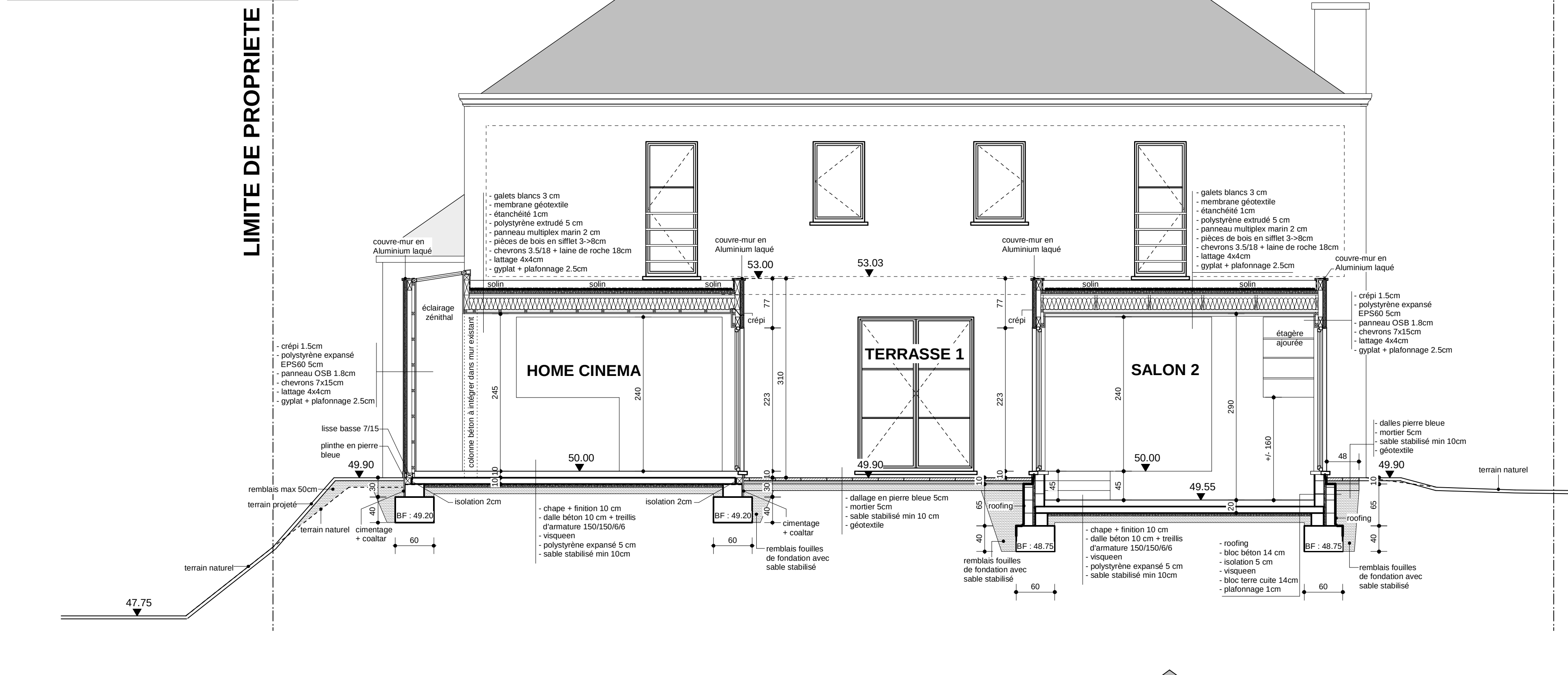
COUPE DD 1/50
