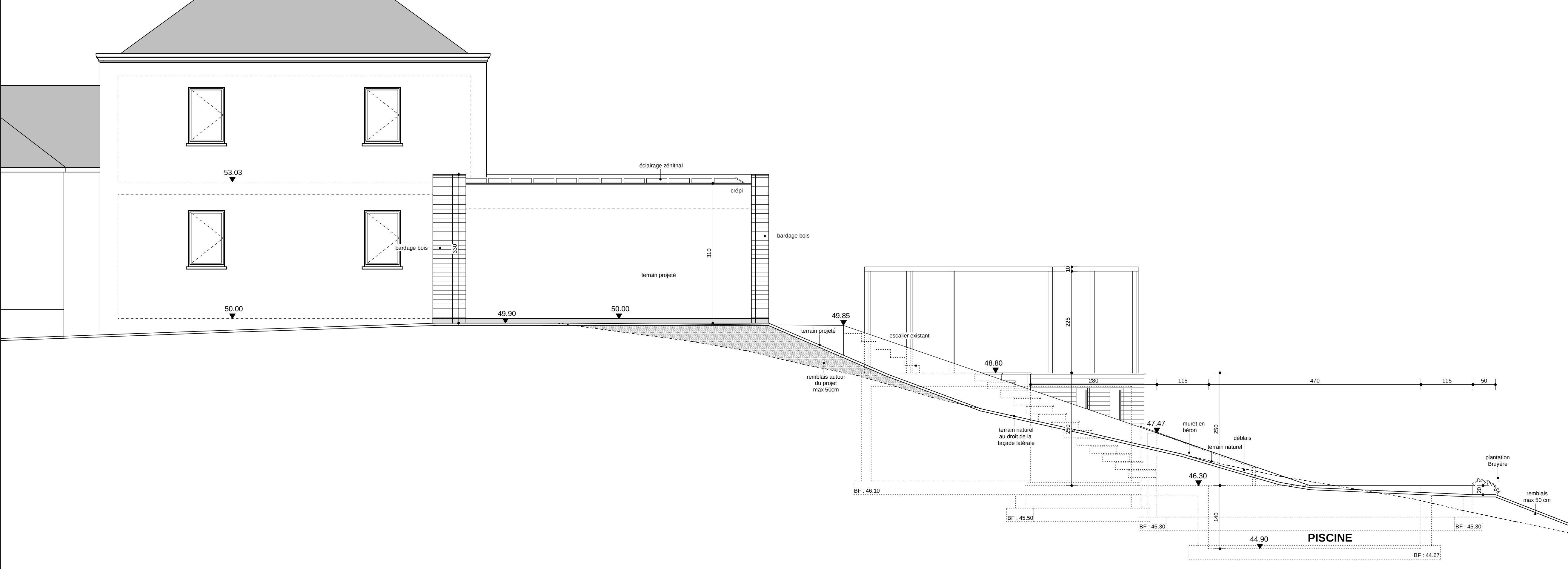
FACADE LATÉRALE DROITE 1/50
