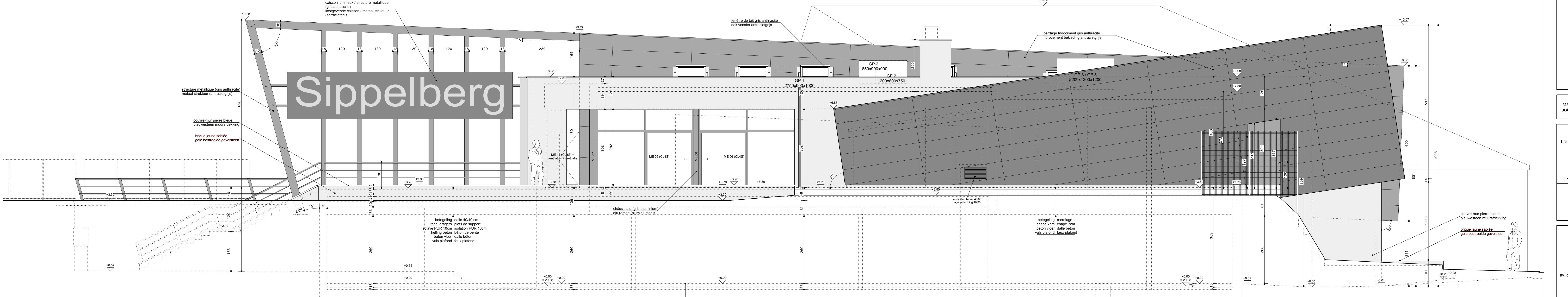
FACADE LATERALE 1/50 ZIJGEVEL 1/50
