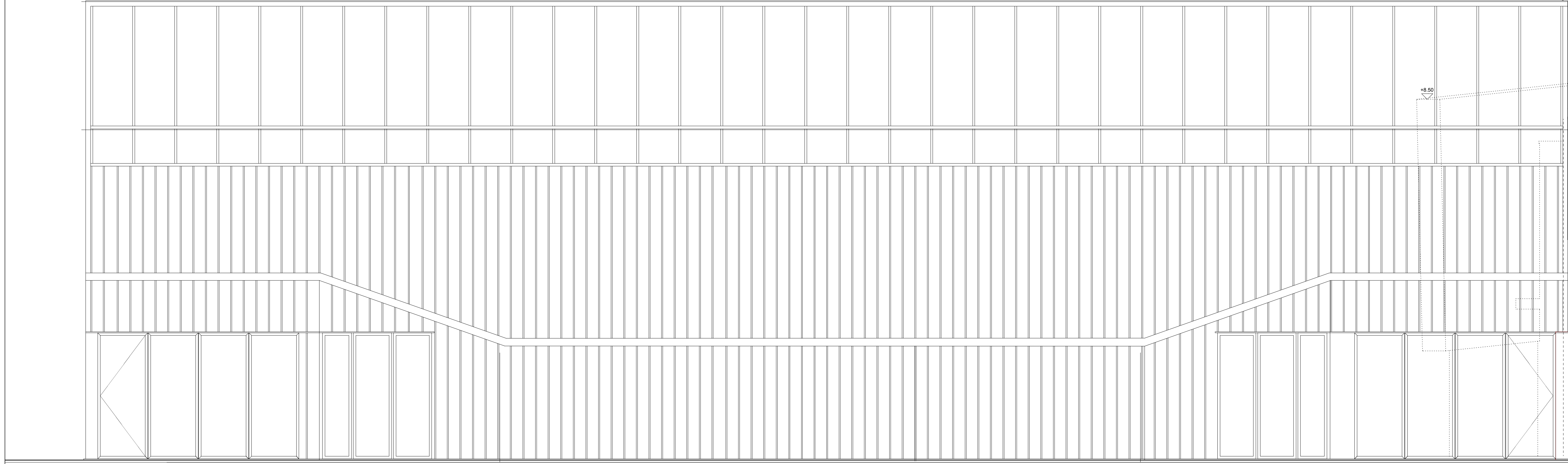
FACADE ARRIERE 2 1/50 ACHTERGEVEL 2 1/50
