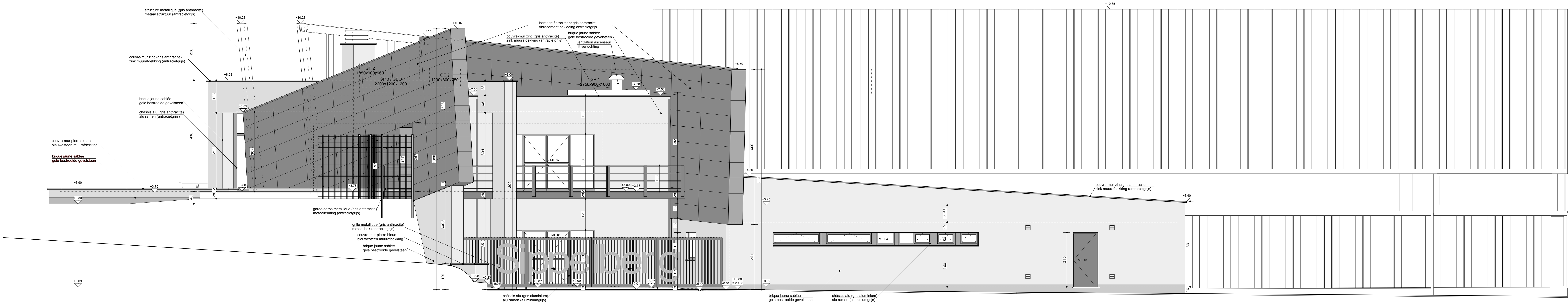
FACADE AVANT 2 1/50 VOORGEVEL 2 1/50
