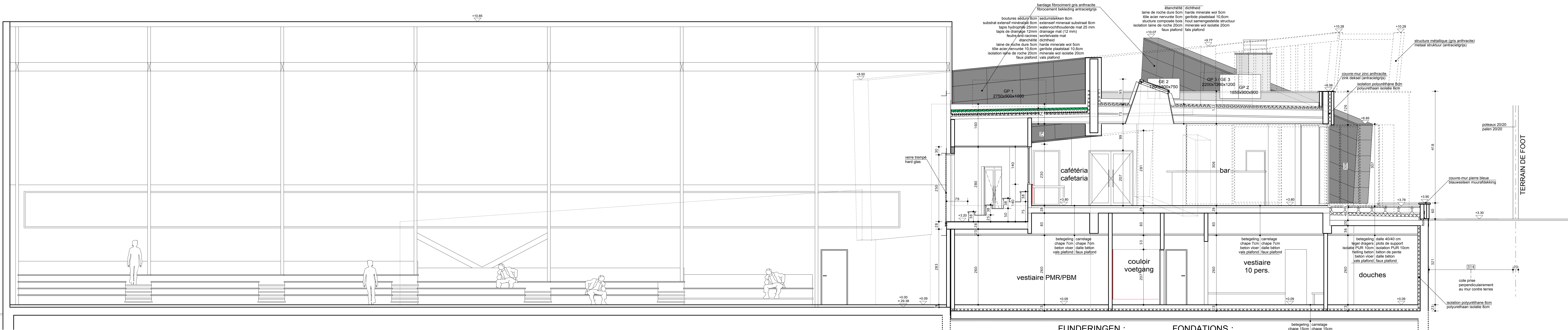
COUPE DD 1/50 DOORSNEDE DD 1/50
