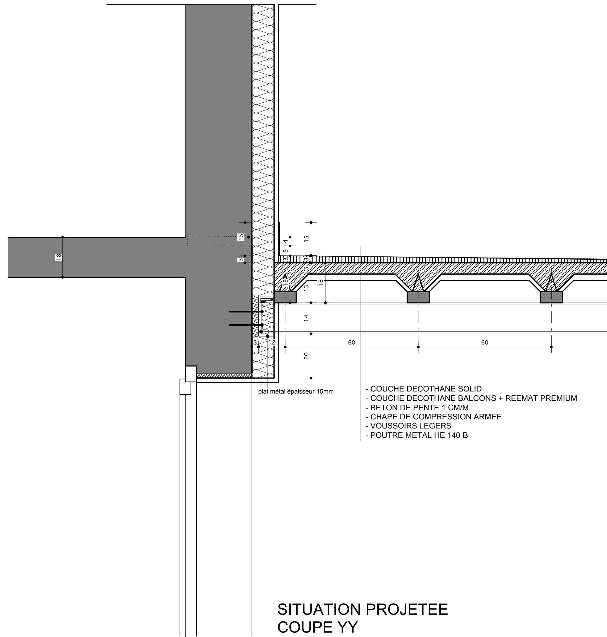
SITUATION PROJETEE COUPE XX
