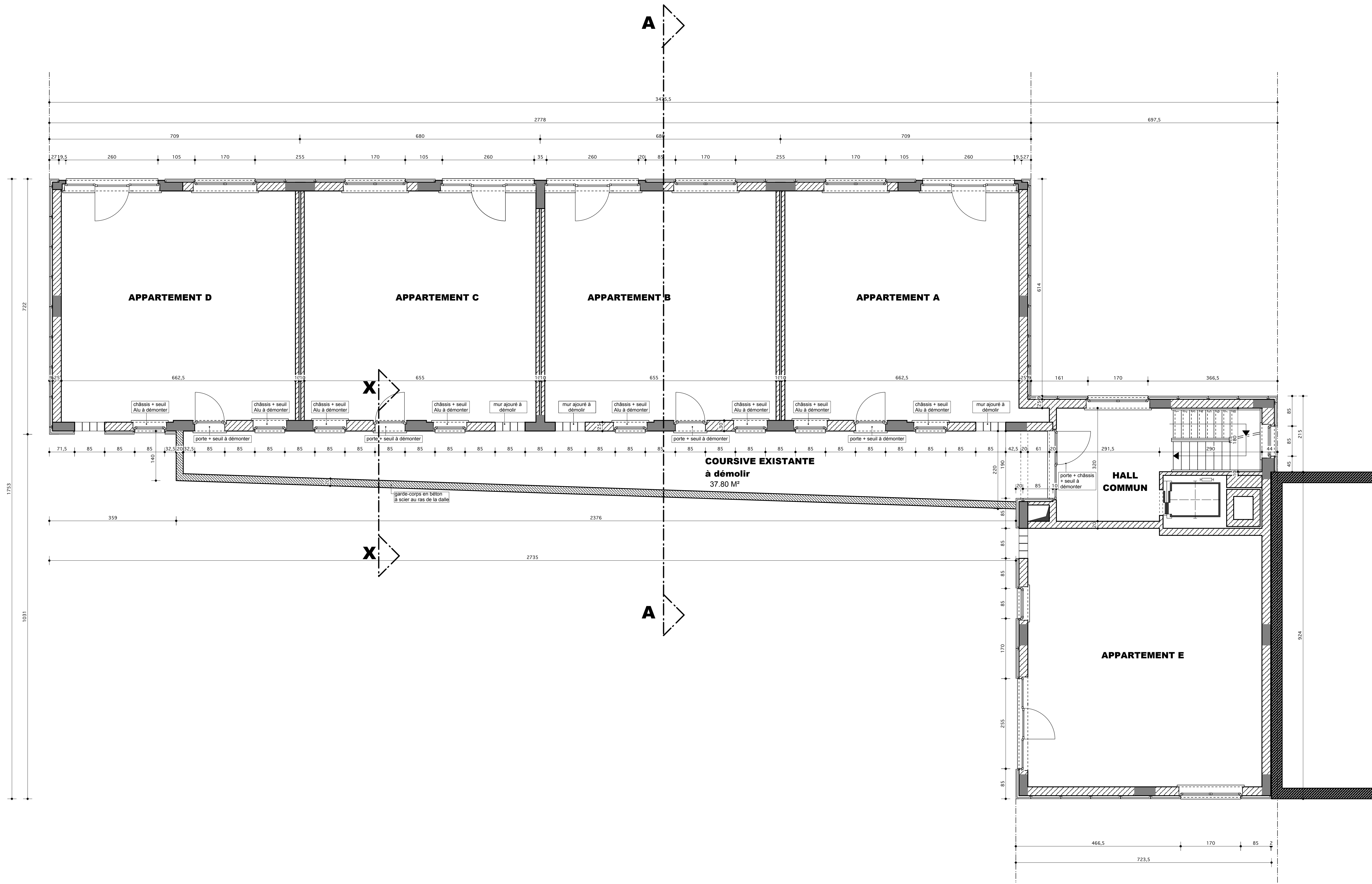
SITUATION EXISTANTE - ETAGE TYPE
