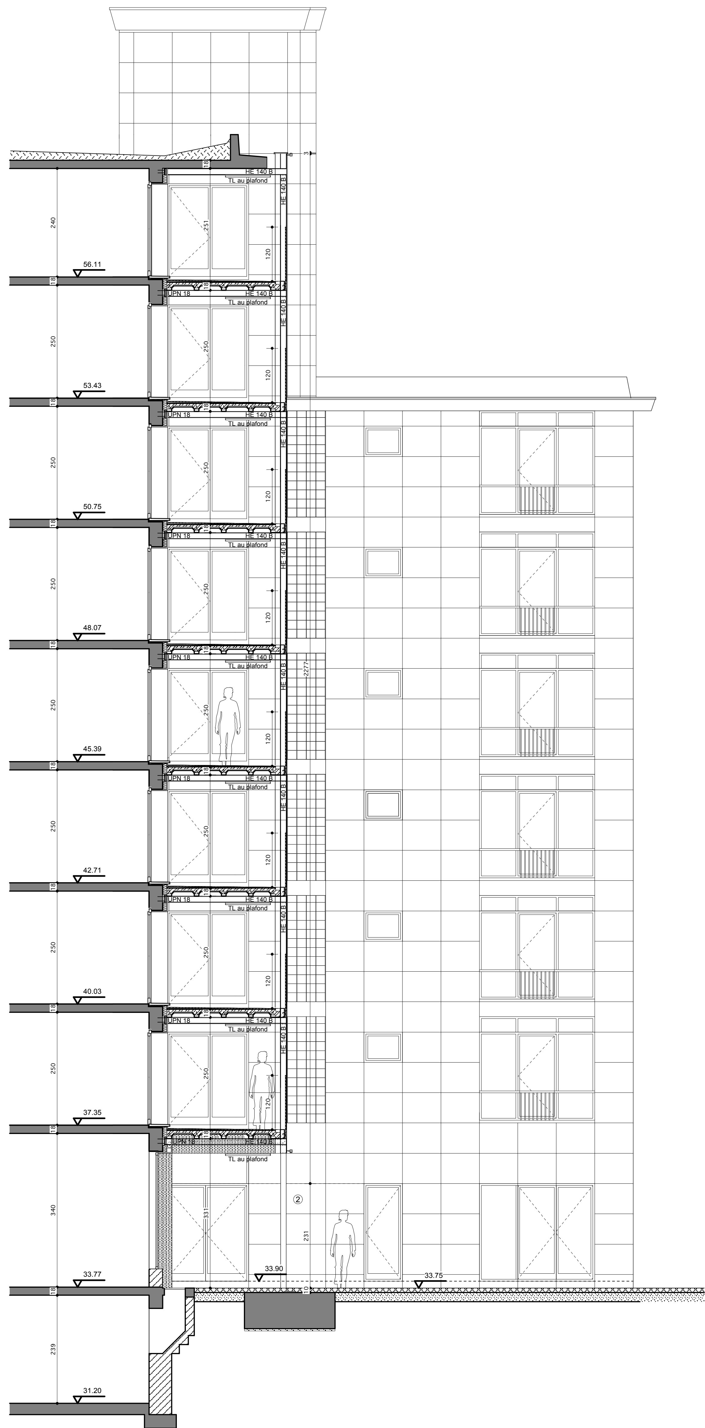
SITUATION PROJETEE COUPE AA
