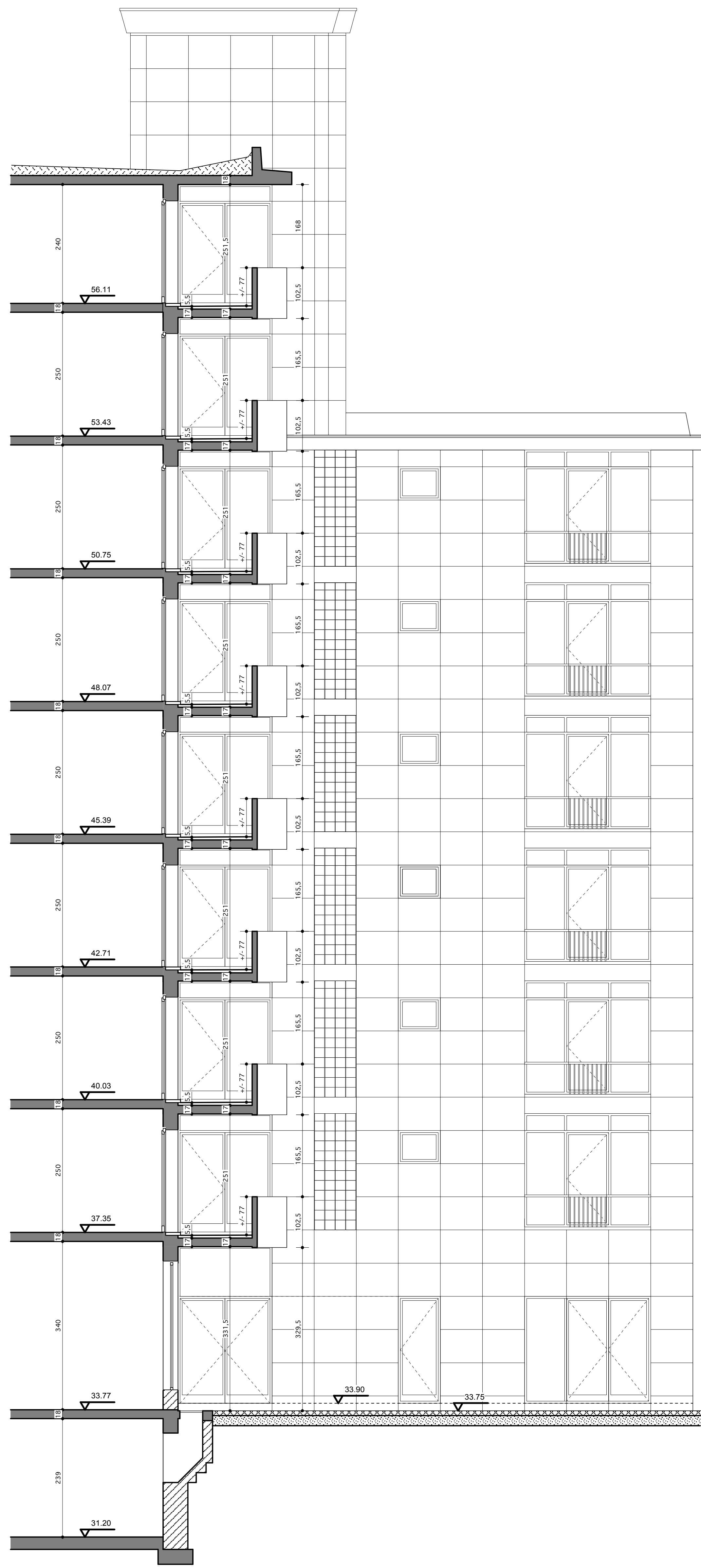
SITUATION EXISTANTE COUPE AA
