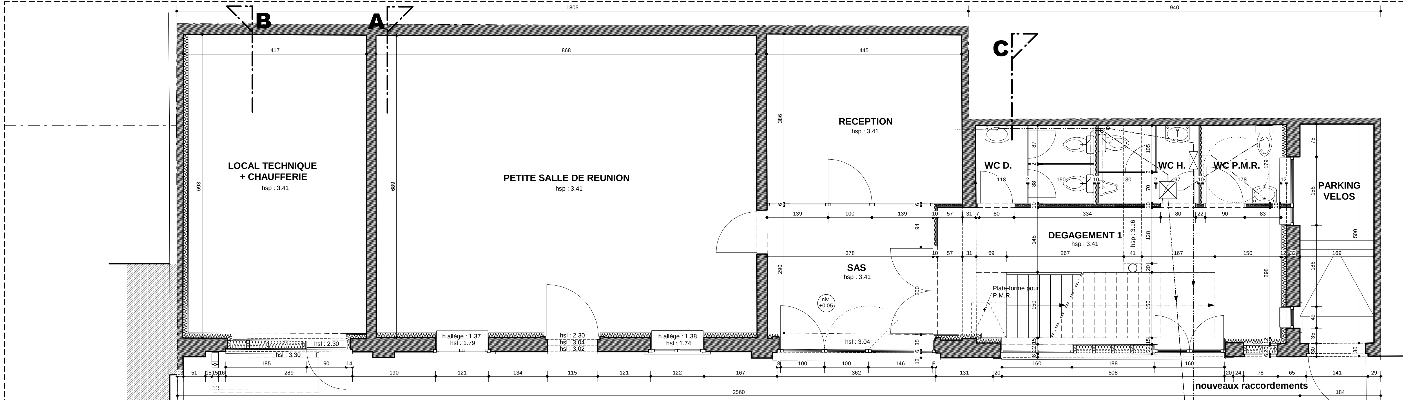
PLAN REZ-DE-CHAUSSÉE
