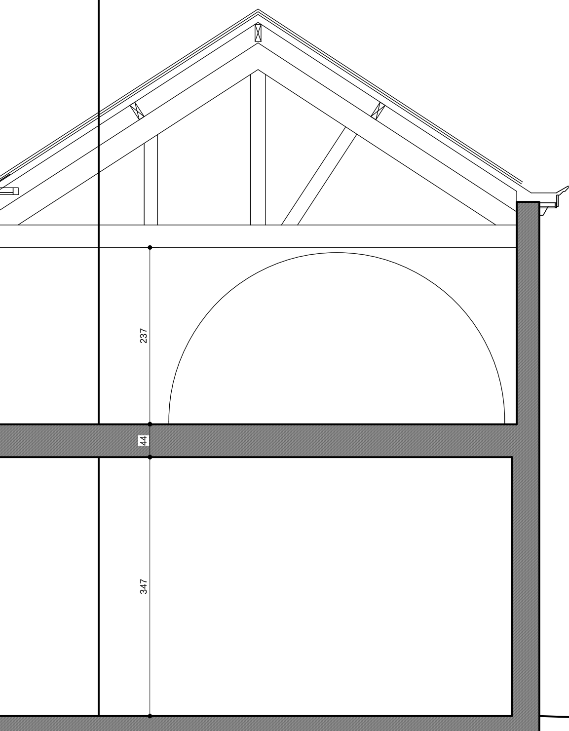
COUPE AA
