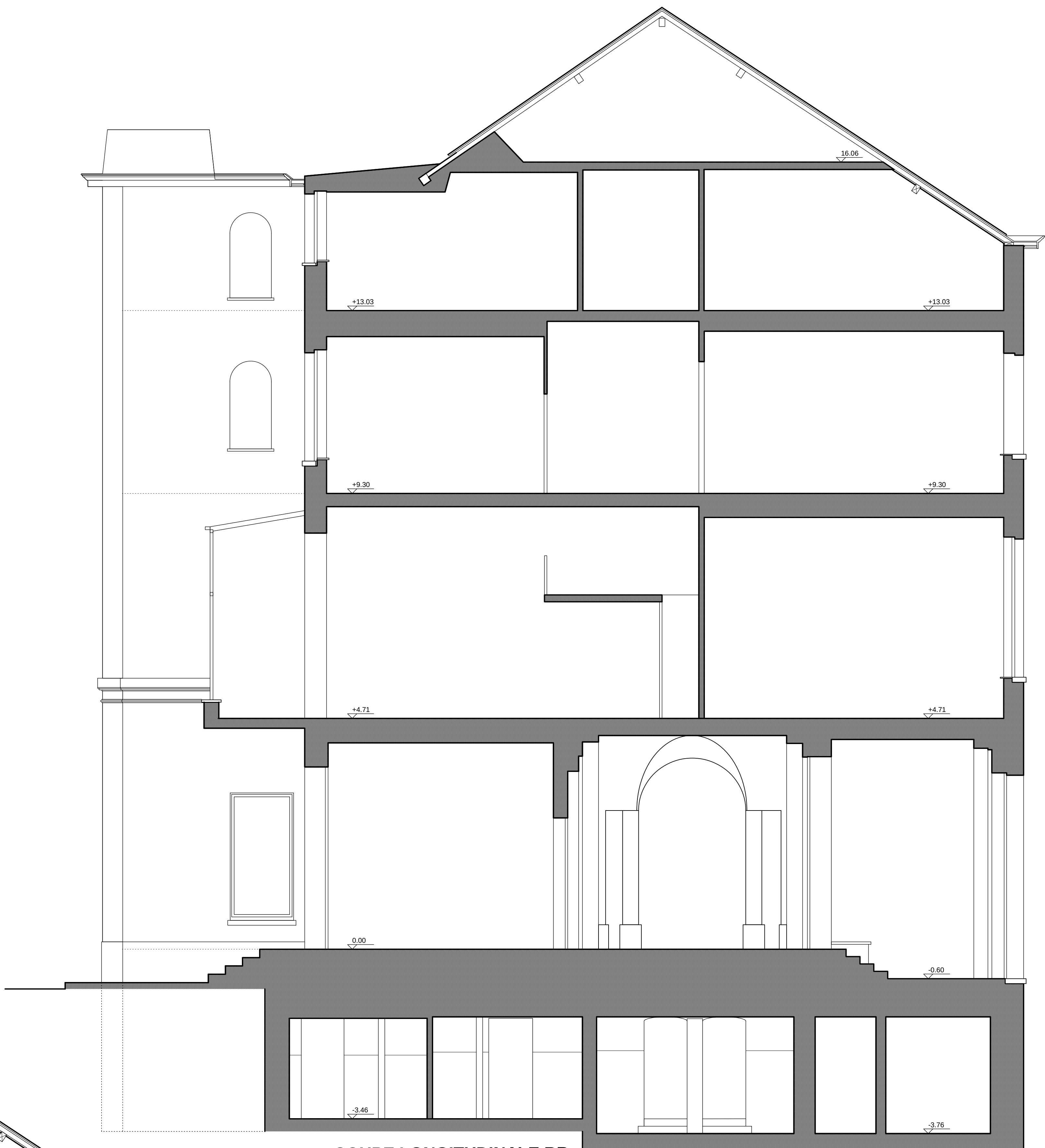
COUPE LONGITUDINALE BB
