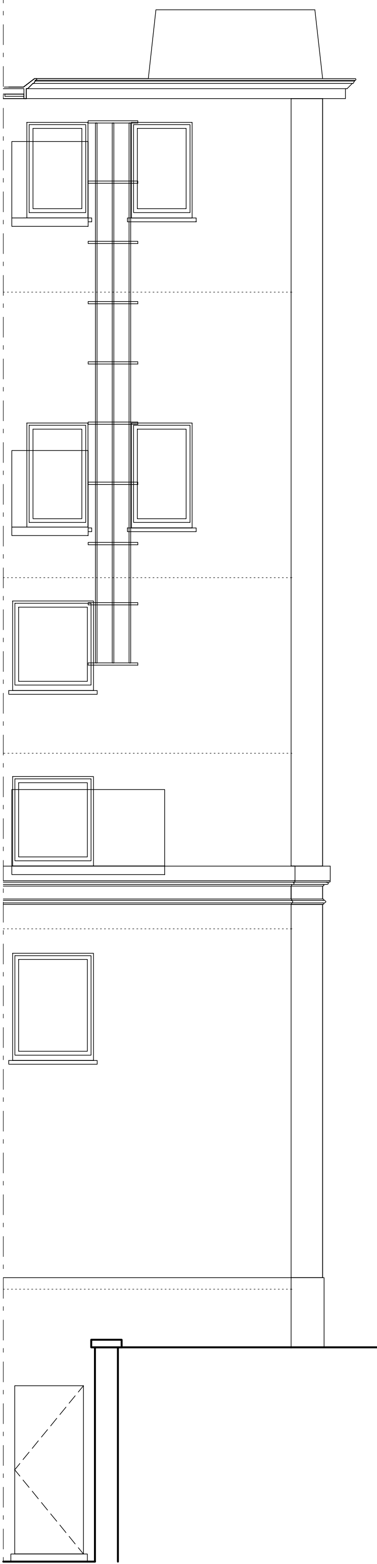
FACADE LATERALE GAUCHE
