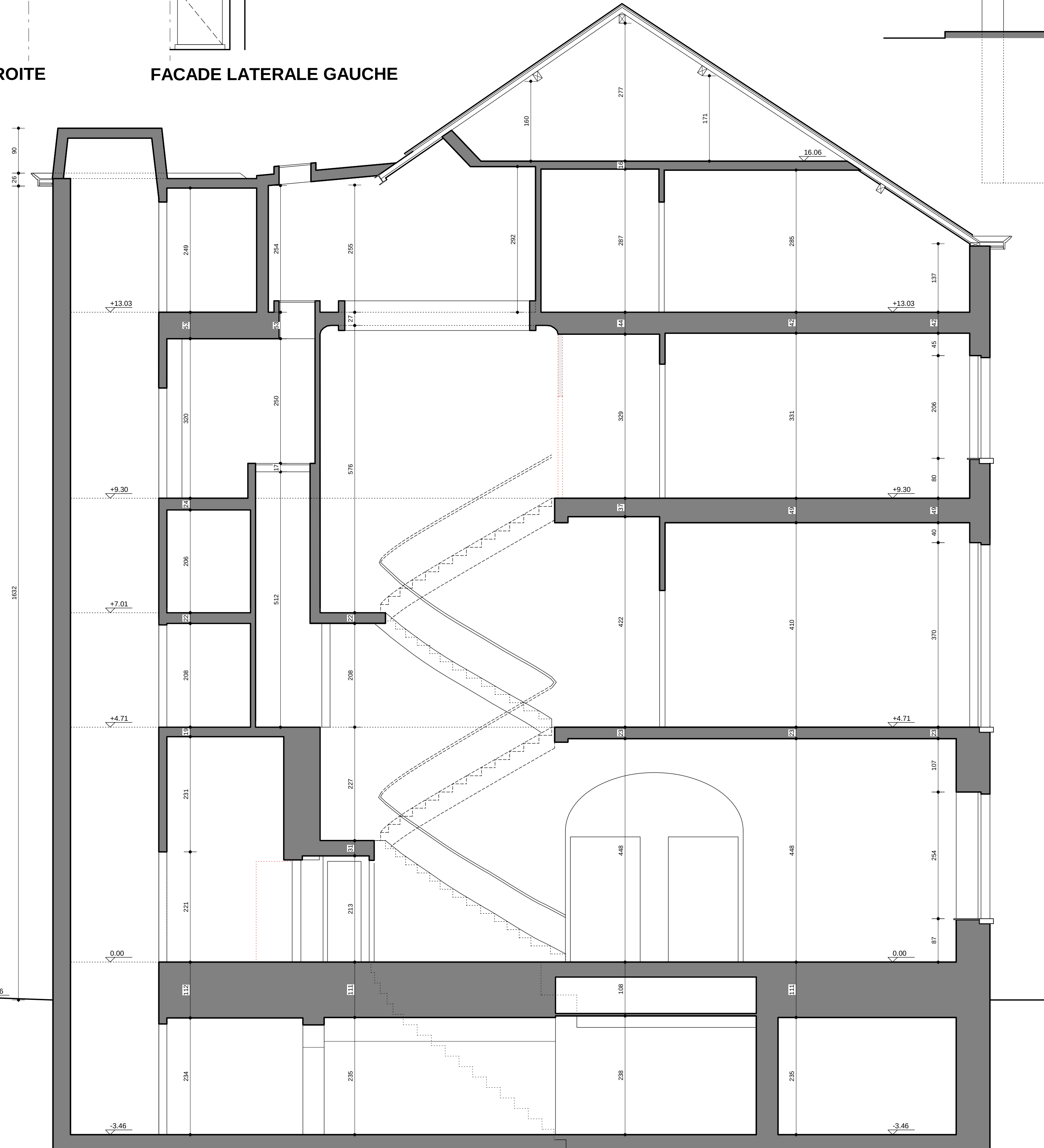
COUPE LONGITUDINALE AA
